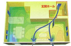
採風ドアの場合
